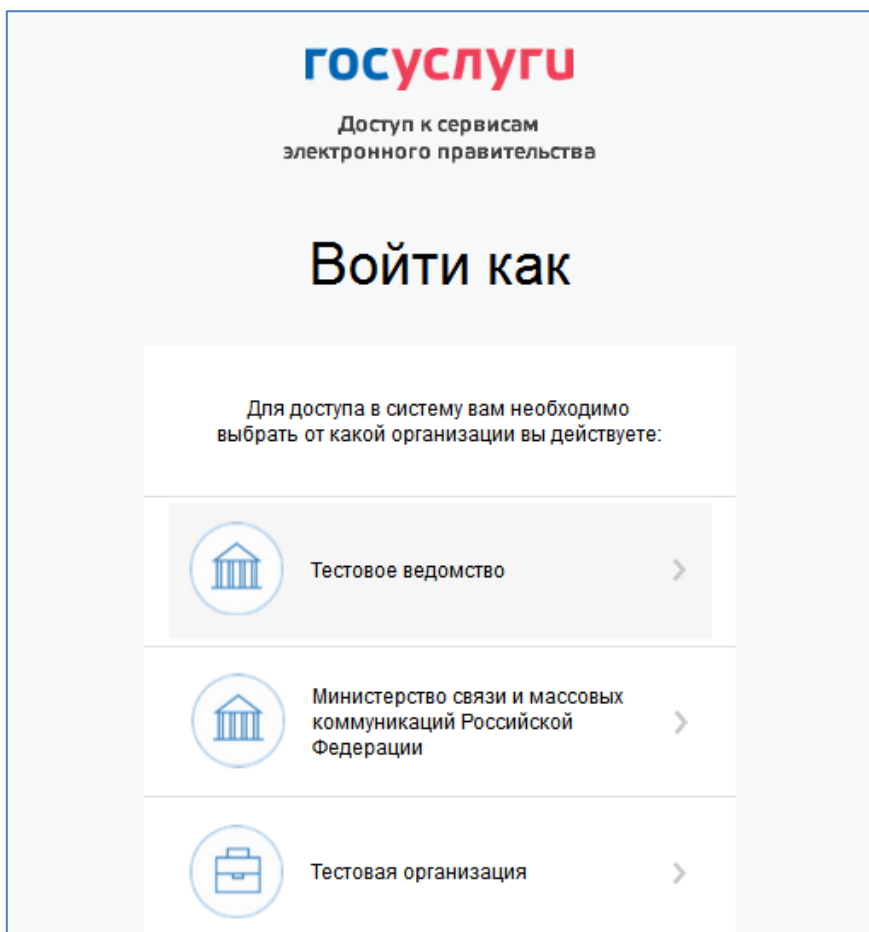
Рисунок 7 – Выбор организации
