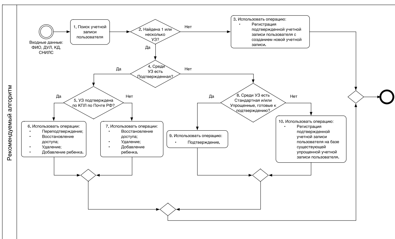
Рисунок 9 – Рекомендуемый алгоритм использования АРМ ЦО
